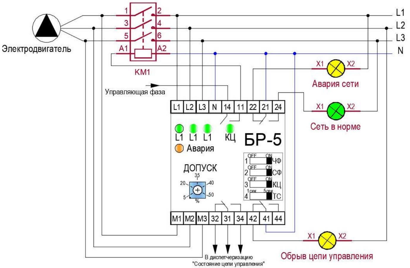
Рисунок 1 – Схема подключений блока «БР-5»
